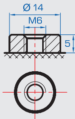
F11 (Schraubanschluss M6)
