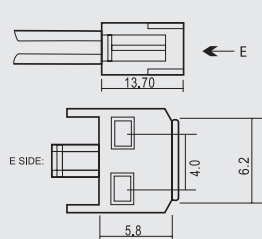
JST-Stecker
