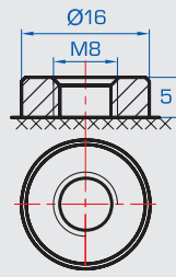
F12 (Schraubanschluss M8)
